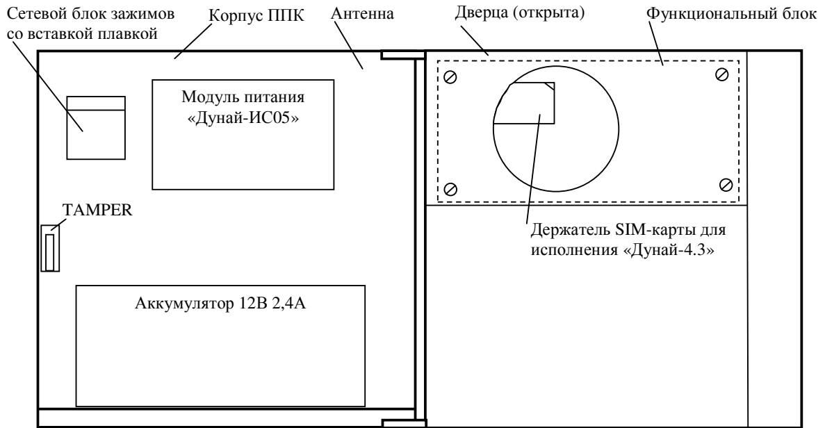
Рисунок В.1 – Размещение модулей в ППК
