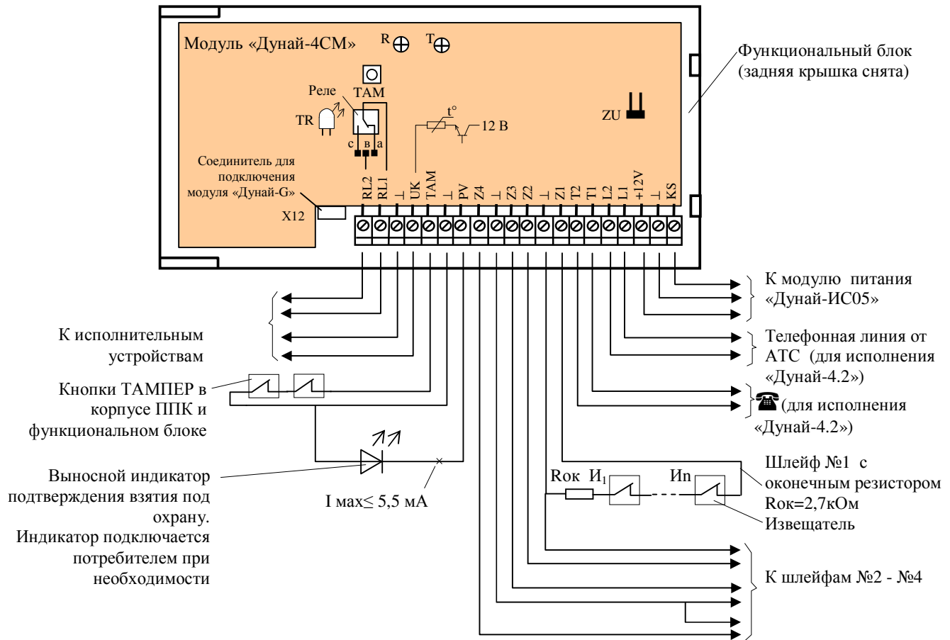
Рисунок Г.1 – Вид модуля «Дунай-4СМ» исполнения «Дунай-4.2»
