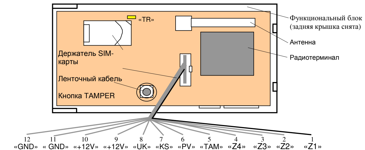
Рисунок Г.1 – Вид модуля «Дунай-4СМ» исполнения «Дунай-4.2»
